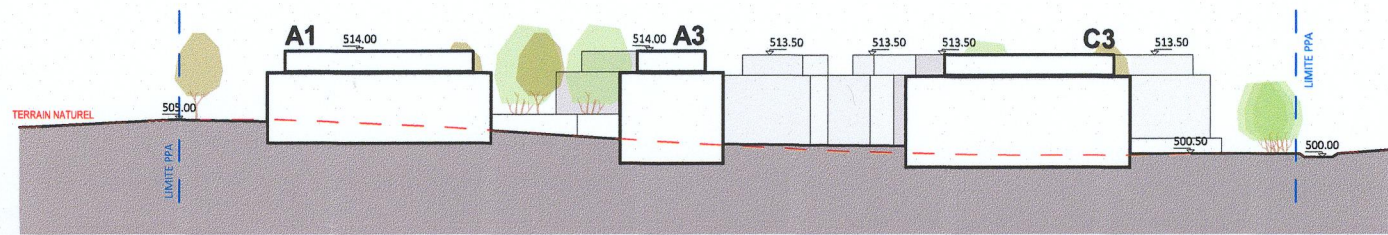
Coupe A-A 1:1000
