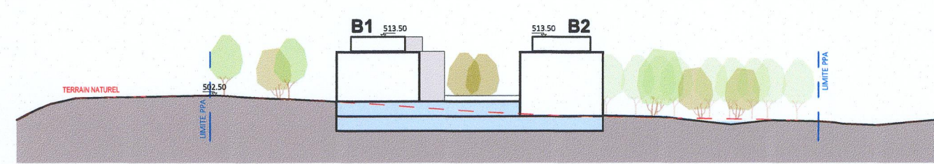
Coupe C-C 1:1000
