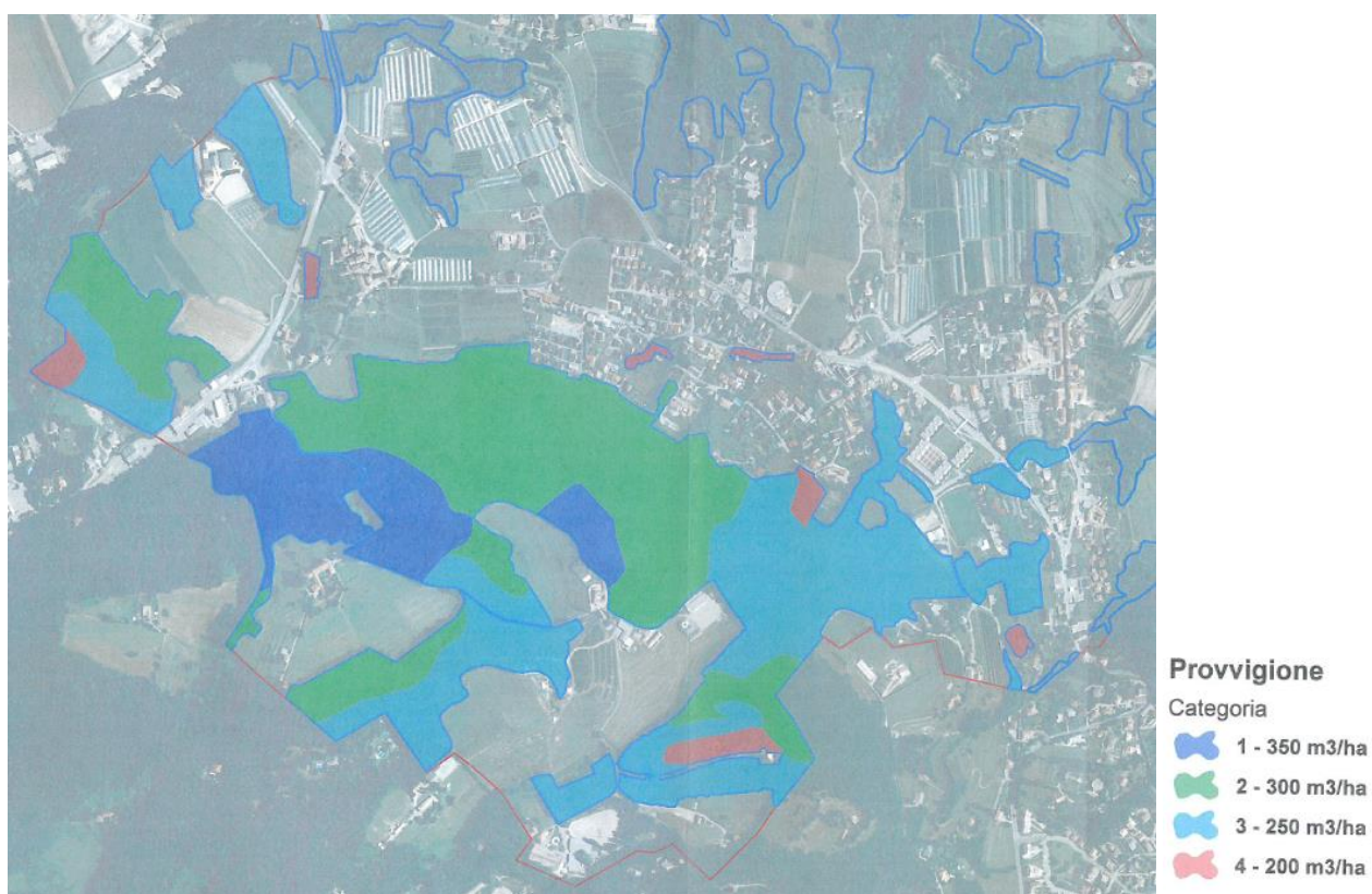
Figura 2: mappa di produttività di approvvigionamento di biomassa legnosa dai boschi comunali.
