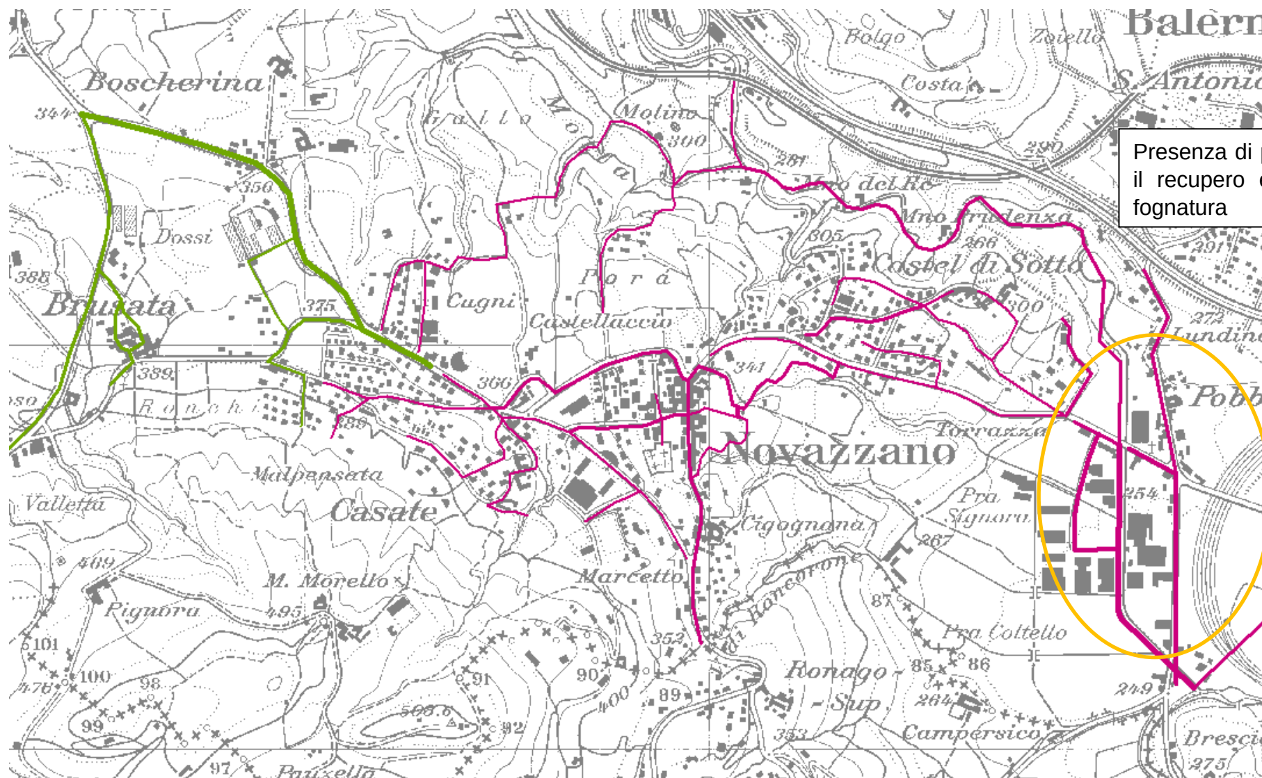
Figura 6: Rete di smaltimento delle acque del comune di Novazzano (la dimensione della linea è proporzionale al diametro del tubo). In verde le canalizzazioni verso il CDA di Mendrisio, in viola le canalizzazioni verso il CDA di Chiasso.
