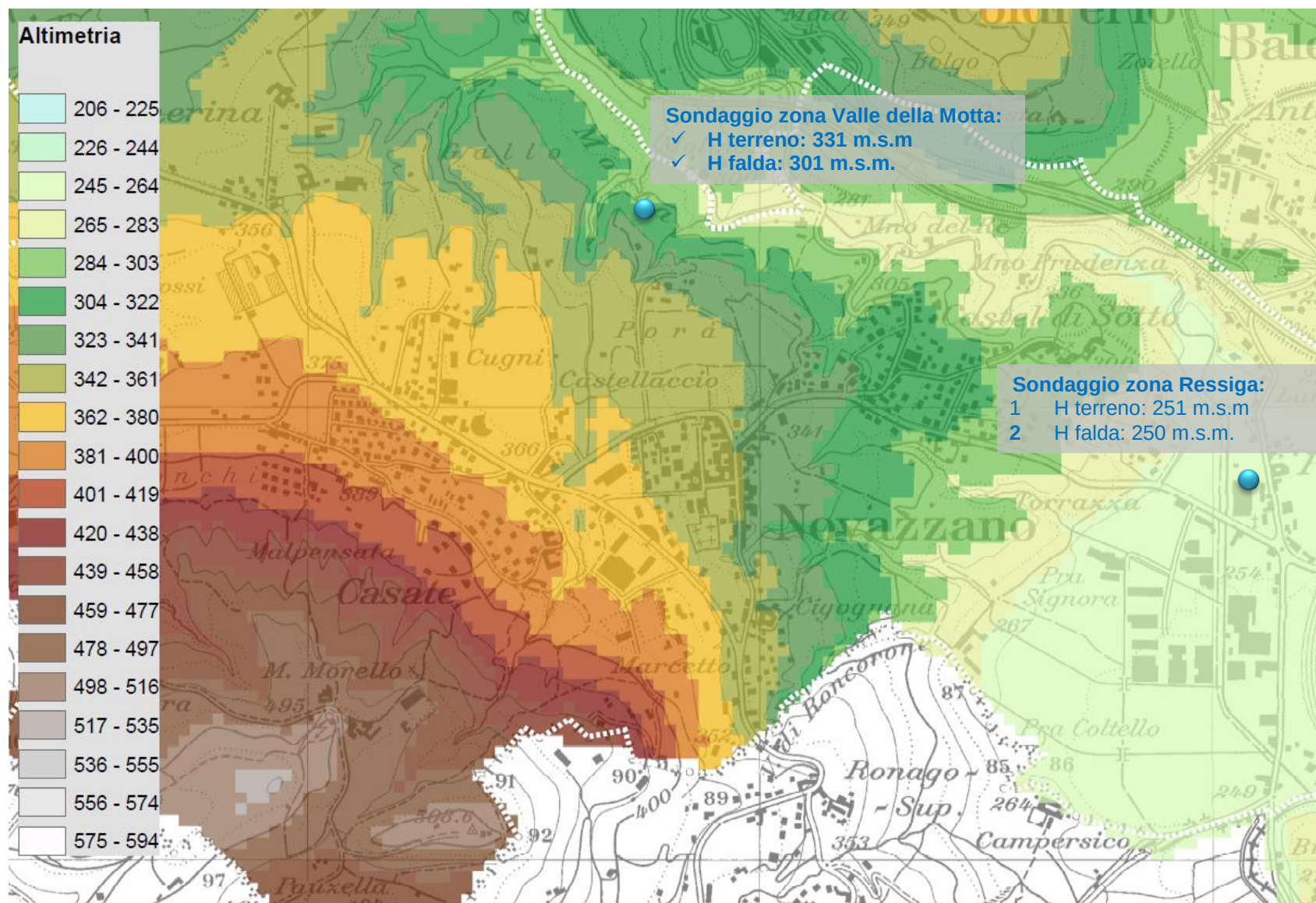
Figura 4: orografia e misurazioni della falda.
