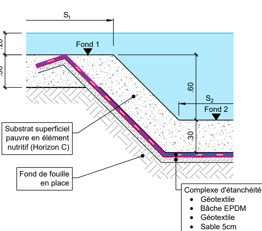
Coupe B - B 1:20 [m]
