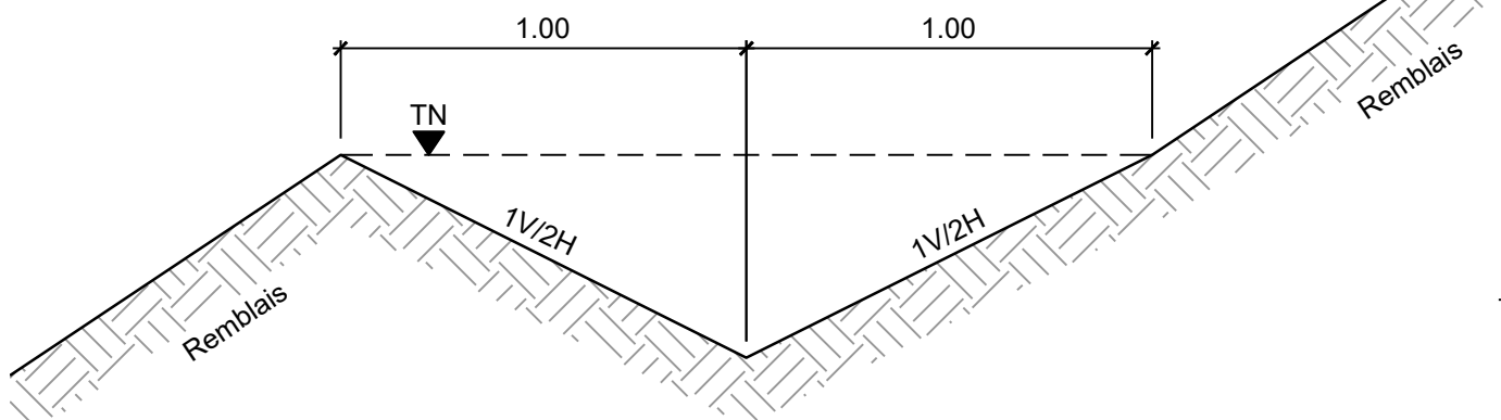
Détail 4 - Chambre de drainage 1:20 [m]
