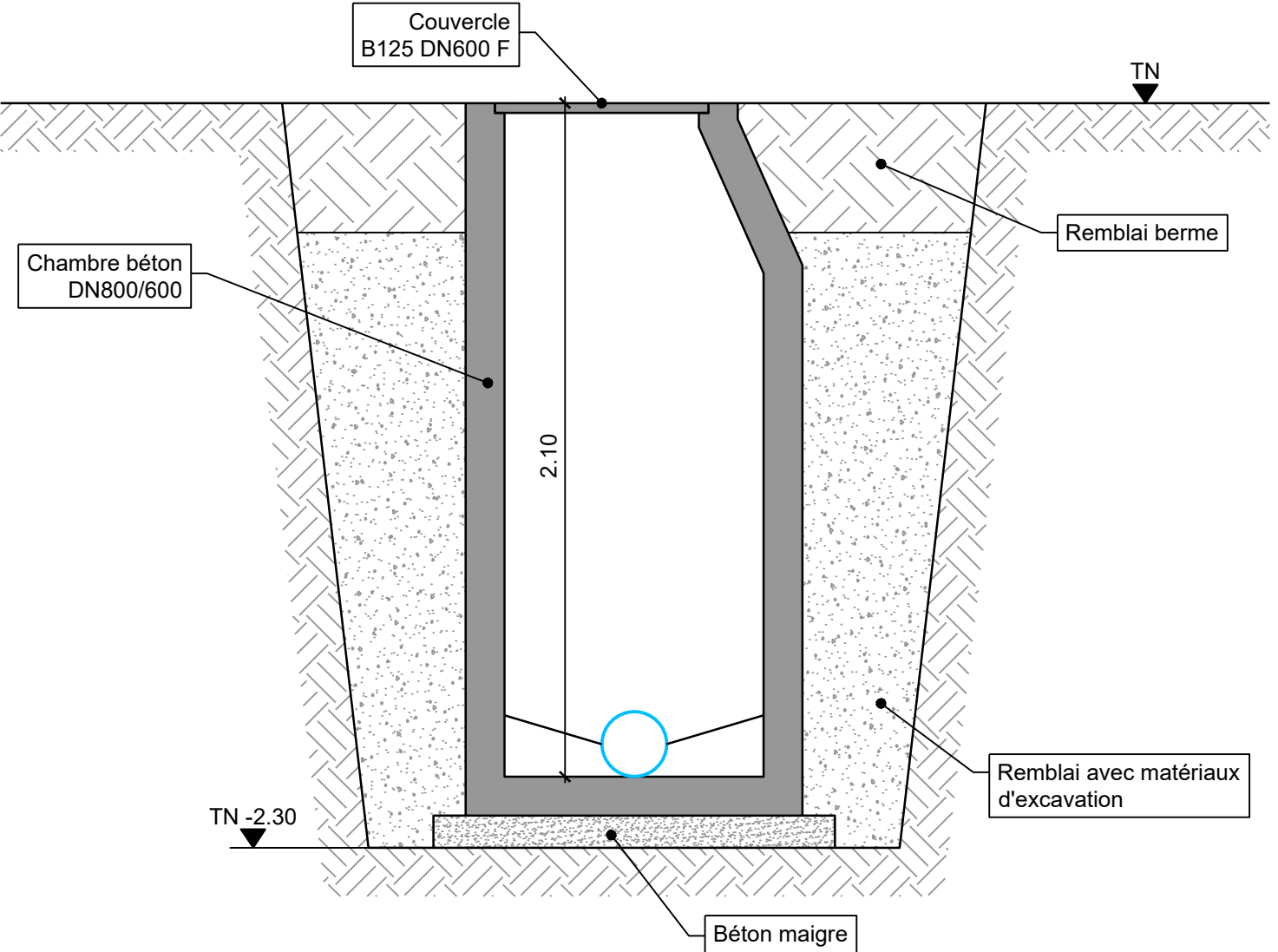
Détail 5 - Coupe type drainage superficiel 1:20 [m]
