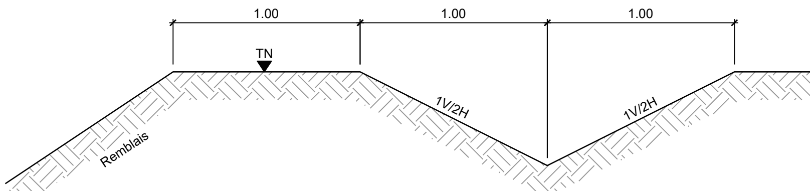
Détail 2 - Fossé de tête de talus 1:20 [m]
