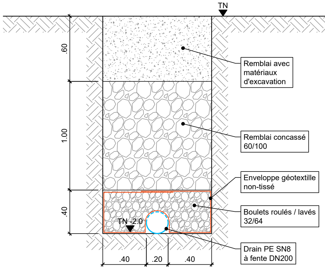
Détail 6 - Coupe type drainage superficiel + profond 1:20 [m]
