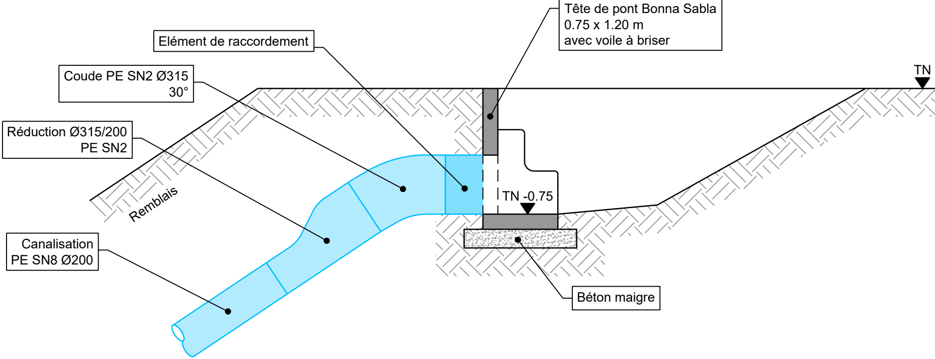
Détail 2 - Fossé de tête de talus 1:20 [m]
