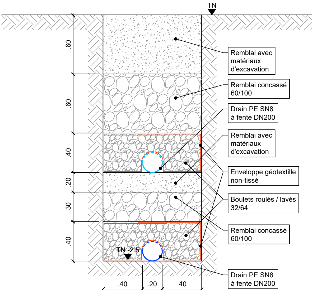
Détail 6 - Coupe type drainage superficiel + profond 1:20 [m]
