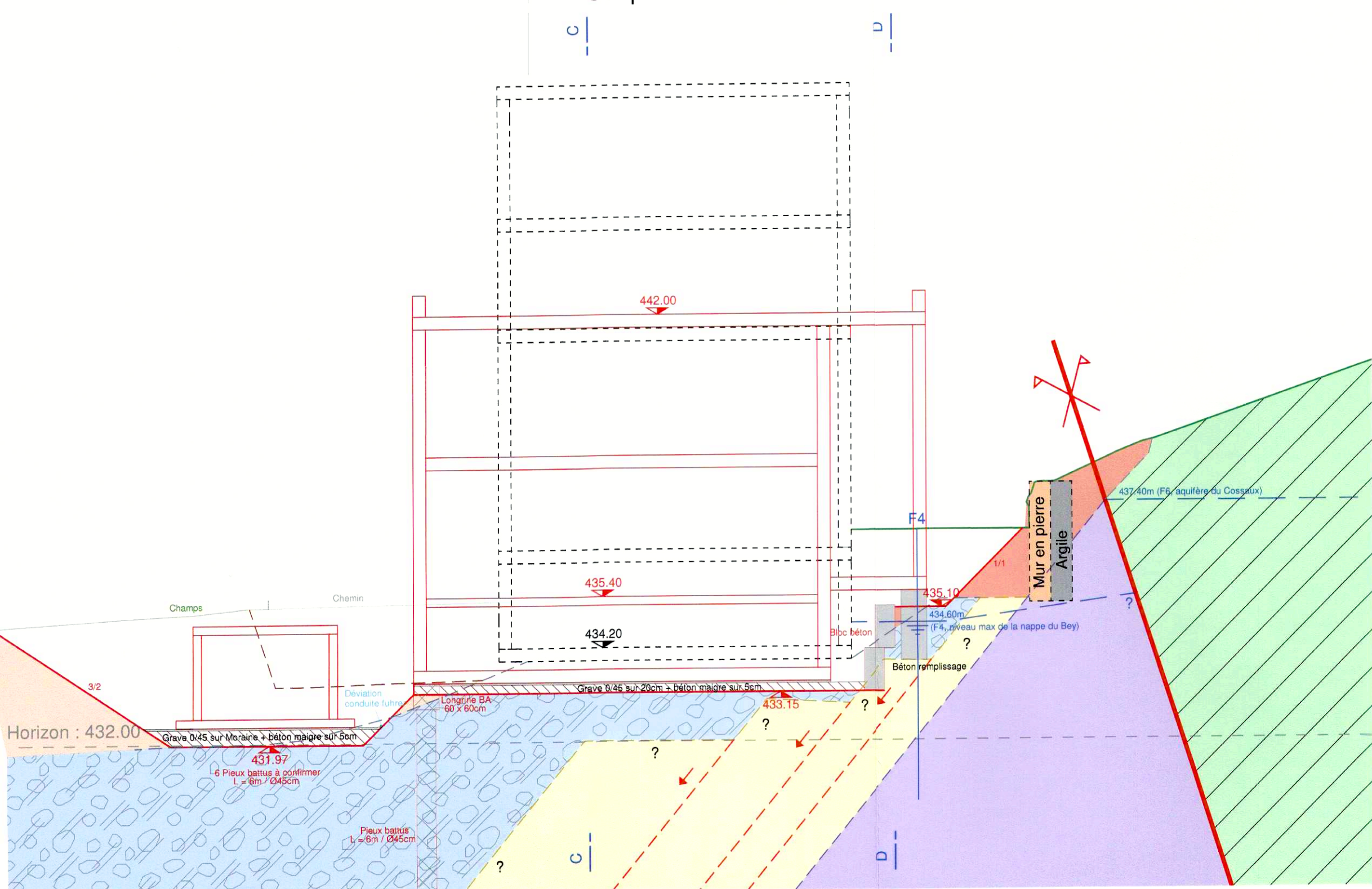
Coupe BB - 1/100
