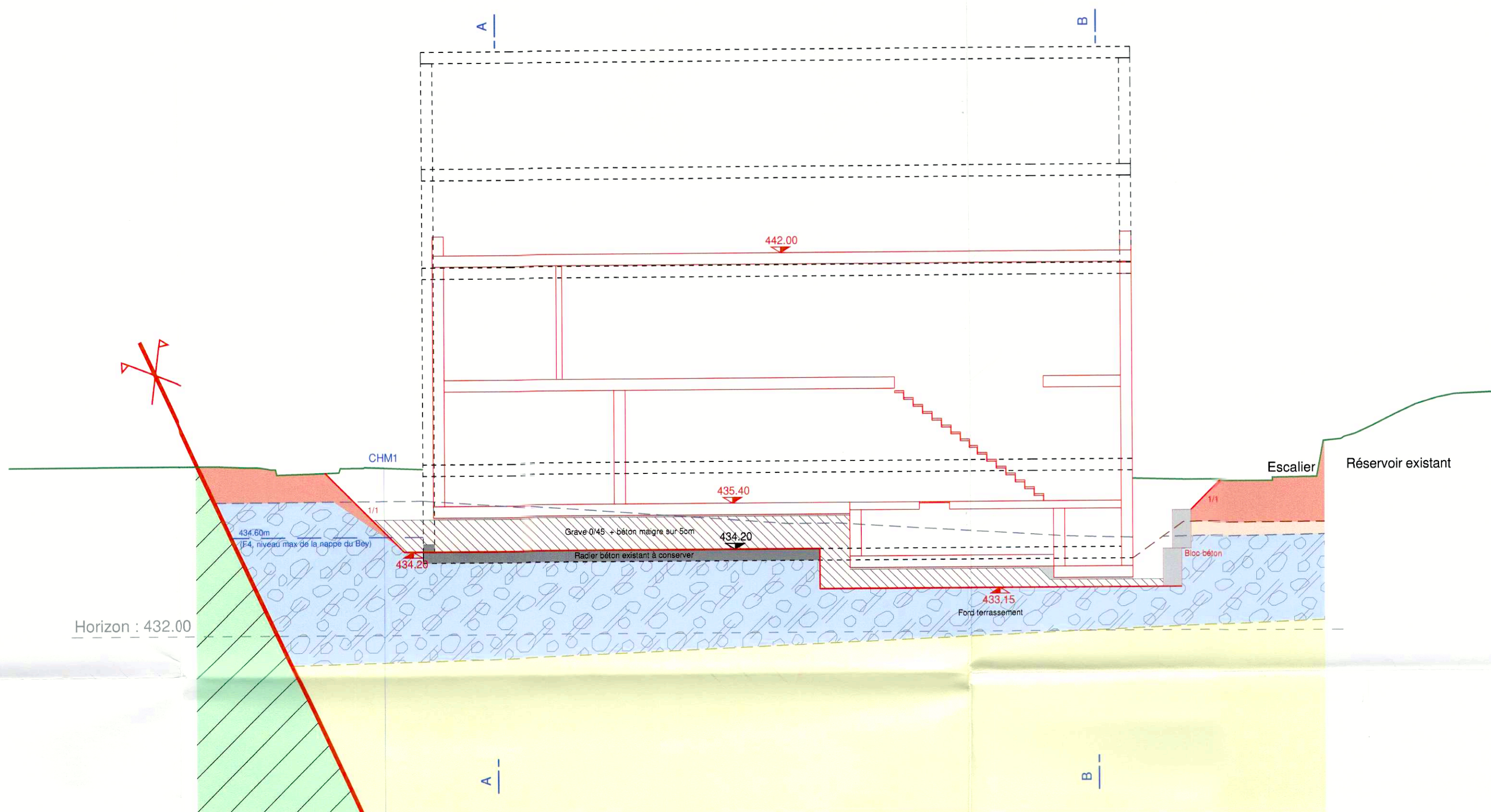
Coupe DD - 1/100
