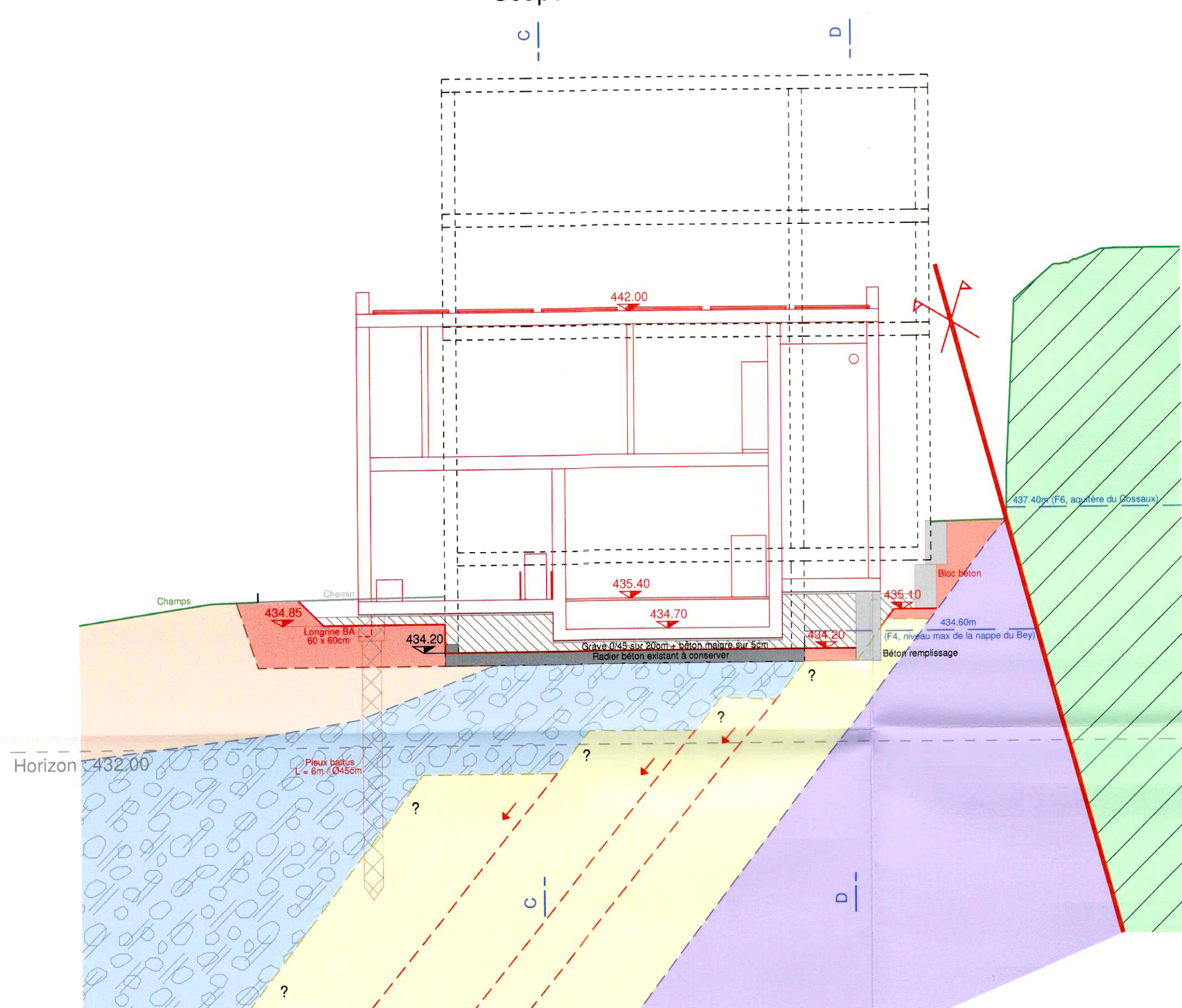
Coupe BB - 1/100
