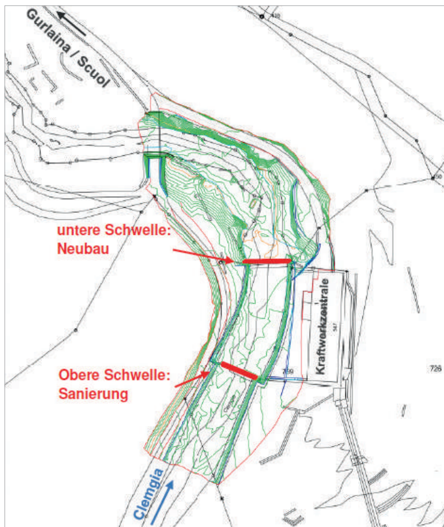
Scuol: Serras pro la centrala da l'ouvra electrica Clemgia
