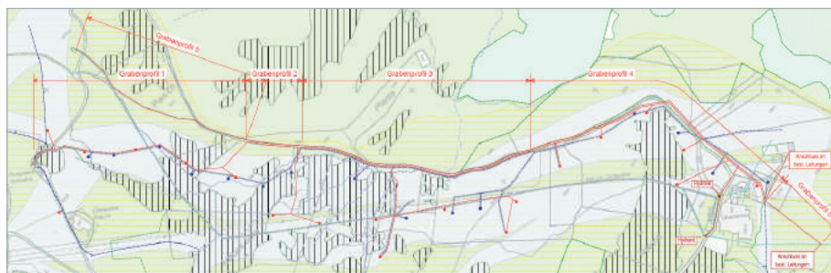
Condot da transport d'aua sü Schlivera/Motta Naluns
