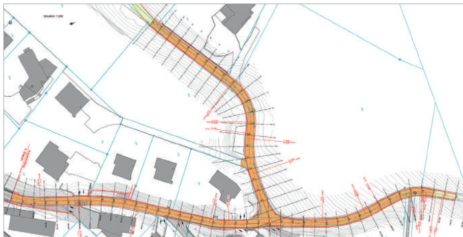
Condots d'aua a Liuns, Scuol
