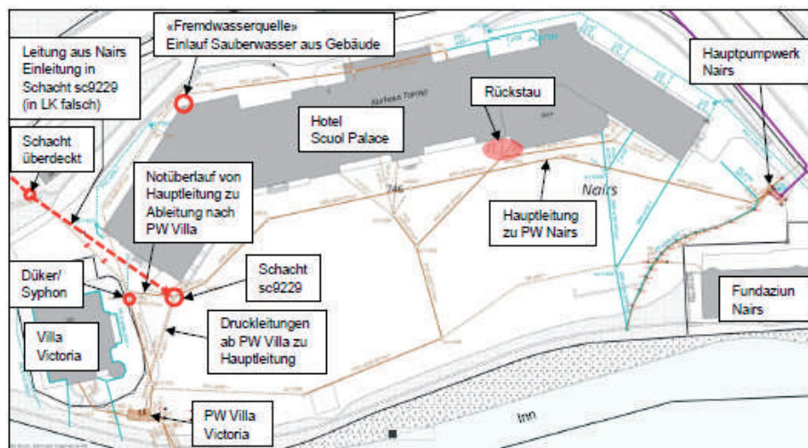
Abbildung 1: Situation im Einzugsgebiet des PW Villa Victoria (Grundlage: Leitungskataster Gemeinde Scuol, Auszug WebGIS vom 18.06.2021)
