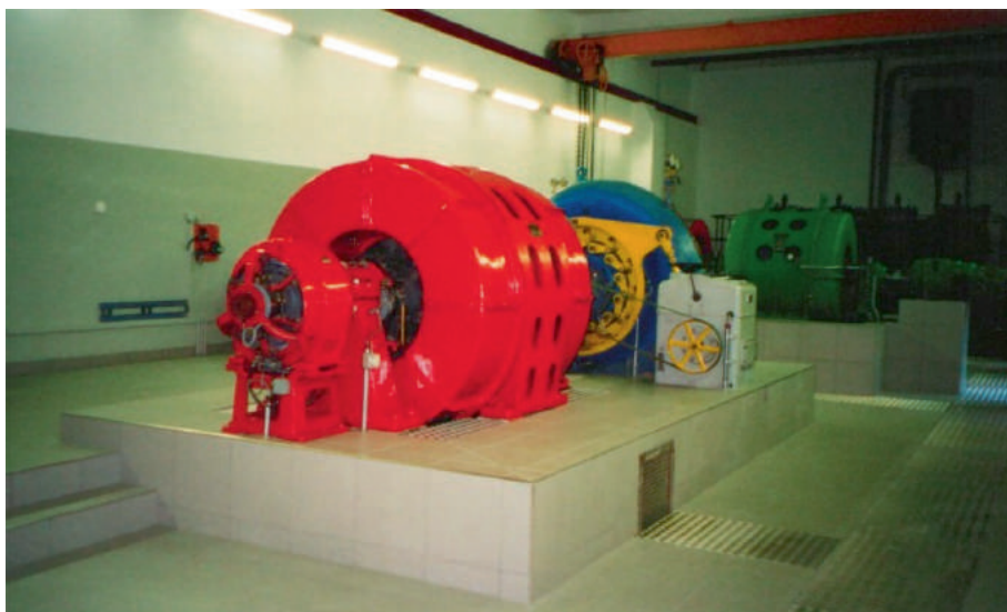
Ouvra electrica Clemgia, Scuol: halla da maschinas
