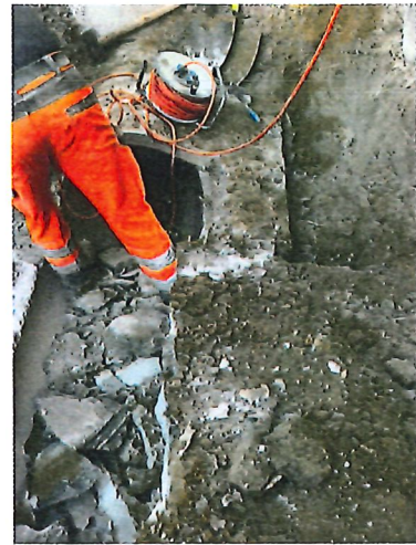
Photo 1 – Epaisseur de l'enrobage non homogène (par endroit double de l'estimation)
