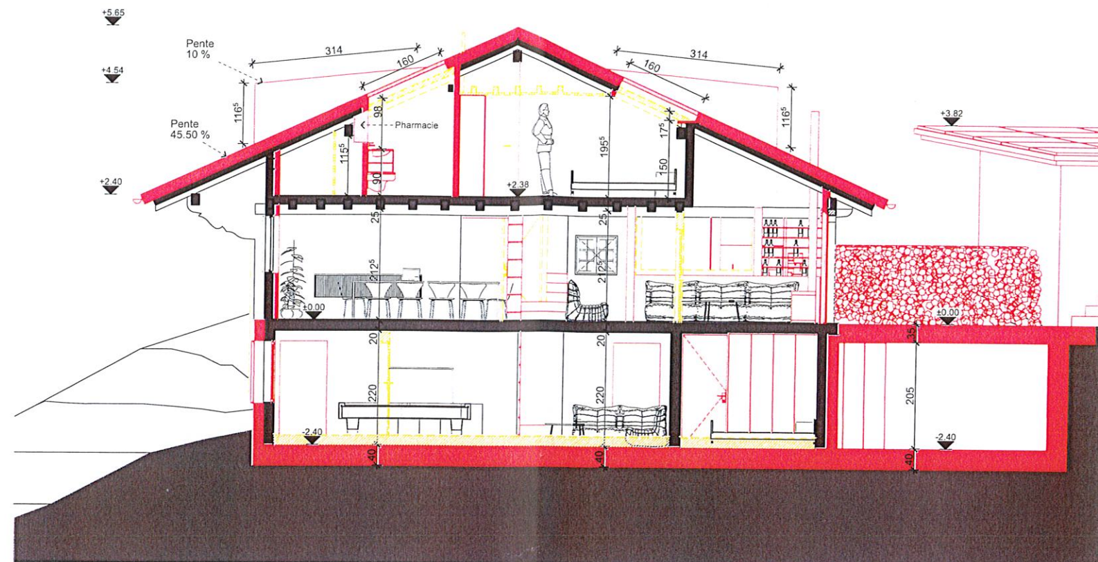
Coupe AA
