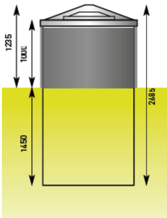
Halbunterflurcontainer
