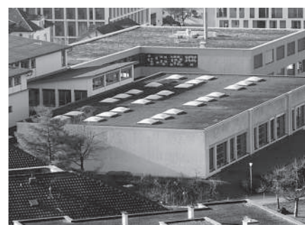
Das Dach der Doppeltturnhalle Haslen ist dringend sanierungsbedürftig
