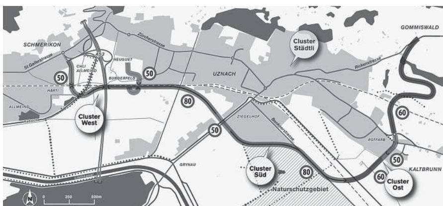
Regionale Verbindungsstrasse, keine Schnellstrasse
