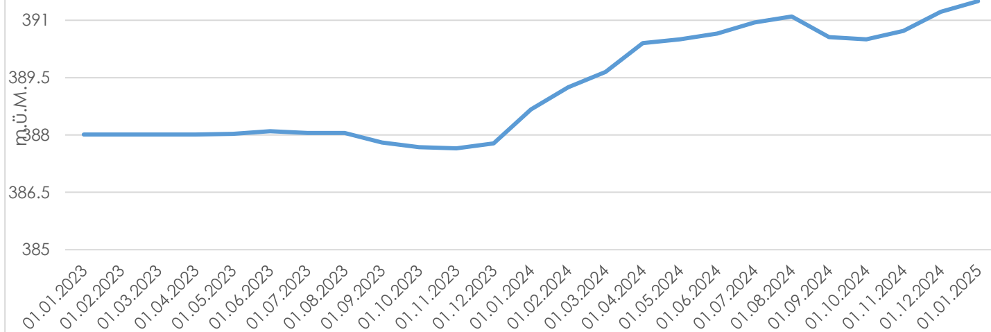
Entwicklung Grundwasserstand
