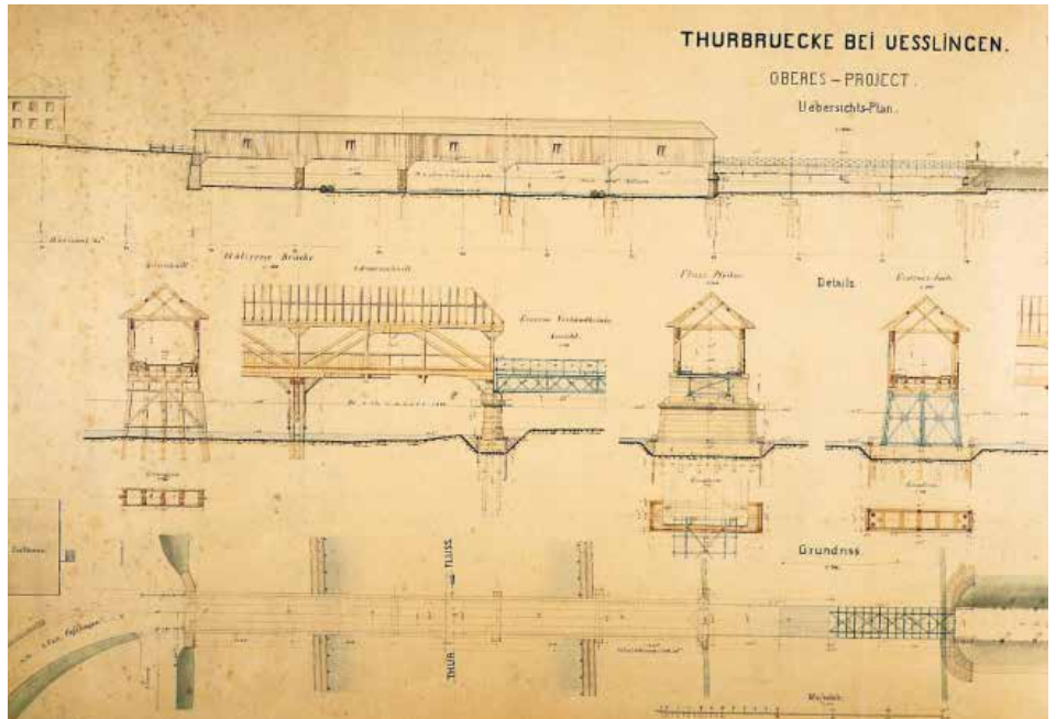
Die Konstruktion der Holzbrücke, erbaut 1808 aufgezeichnet anlässlich des Projektes von 1890
