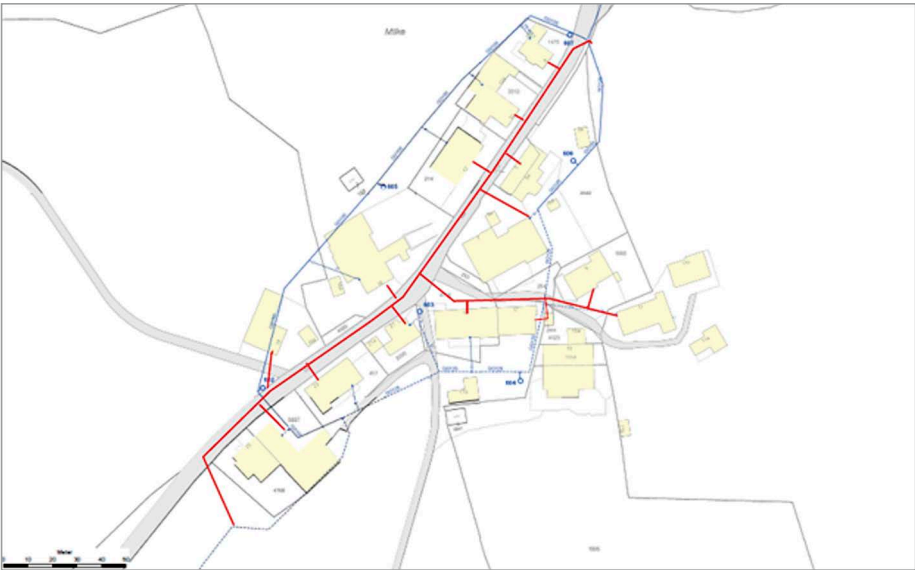
Die alte Wasserleitung Milken Ost und West (blau) soll durch eine neue Leitung (rot) ersetzt werden.
