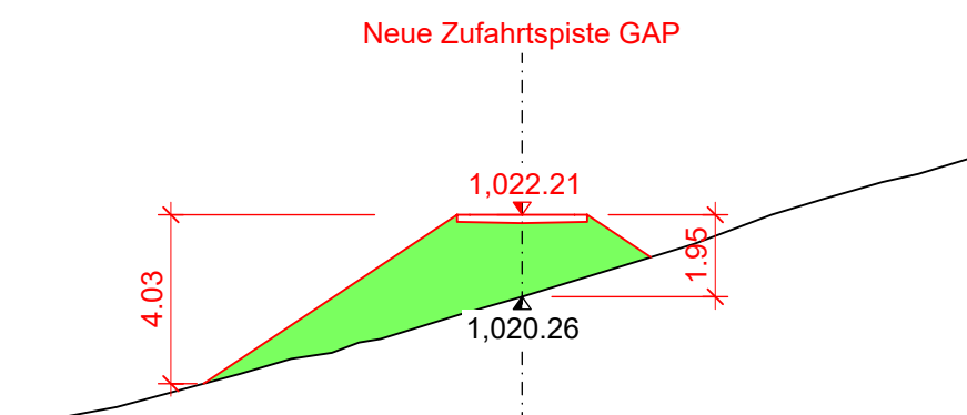
QP 2 1:200
