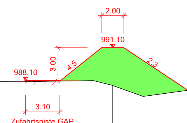
QP Damm 1:200
