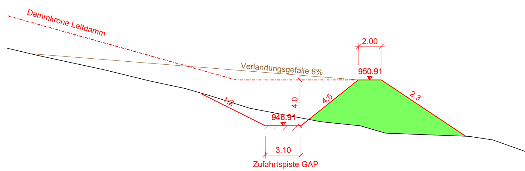
LS Damm 1:200
