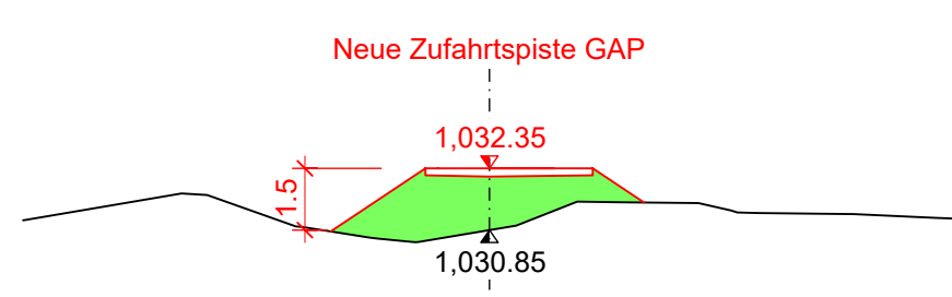
QP 1 1:200
