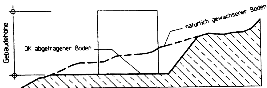
Abb. 6: Gebäudehöhe abgetragen
