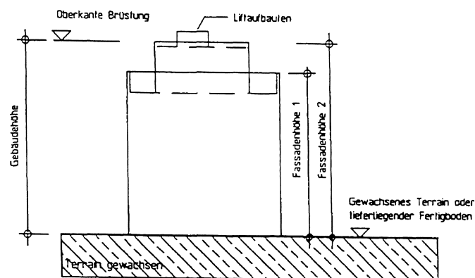
Abb. 8: Höhen am Flachdach
