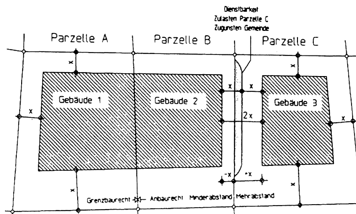
Abb. 5: Ungleiche Grenzabstände
