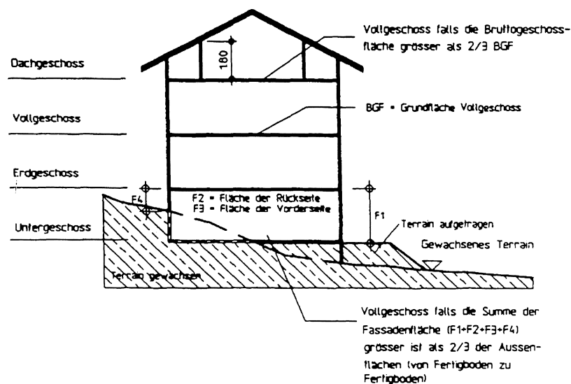
Abb. 11: Geschosse (Satteldach)
