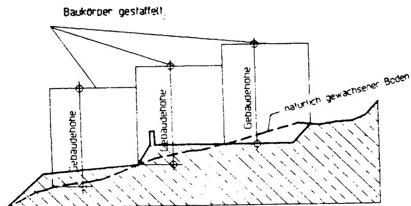
Abb. 10: Gebäudehöhe, Terrain gestaffelt
