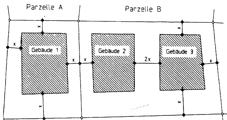
Abb. 4: Grenz- und Gebäudeabstand
