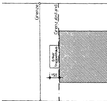
Abb. 2: Grenzabstand bei auskragenden Bauteilen, Normalfall
