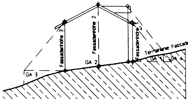
Abb. 1: Grenzabstand in Abhängigkeit der Fassadenhöhe
