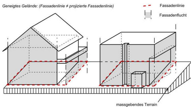
Abbildung 1: Figur 3.1 bis 3.3 Fassadenflucht und Fassadenlinie, IVHB
