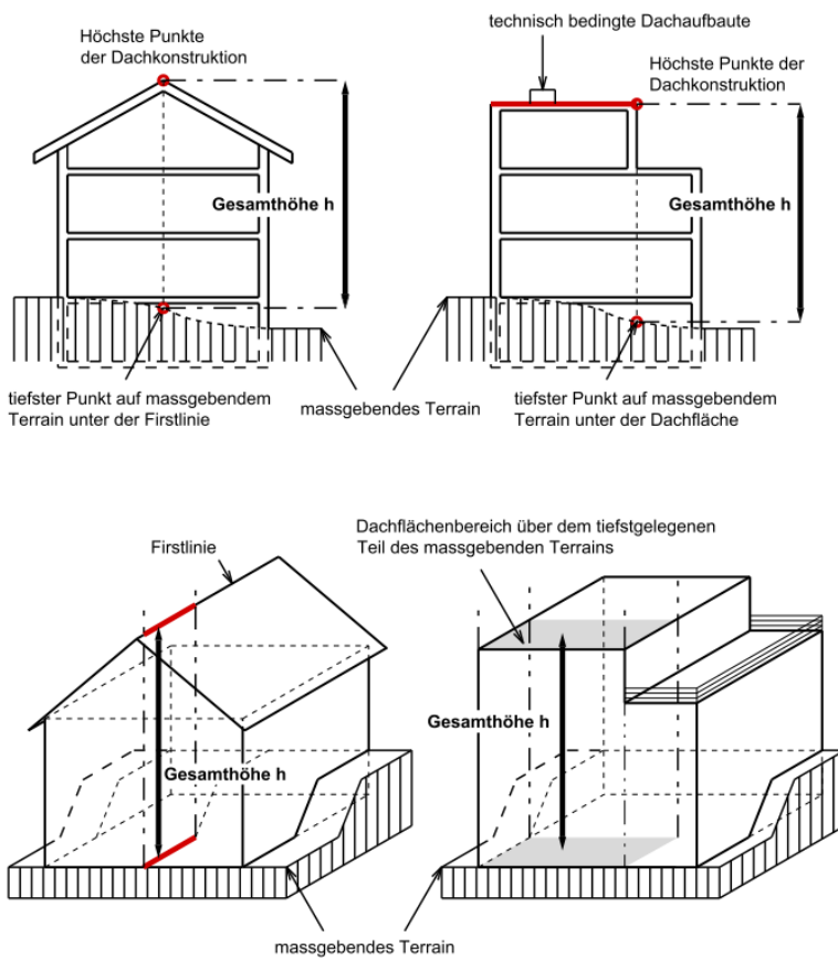
Abbildung 10: Figur 5.1 Messweise Gesamthöhe, IVHB
