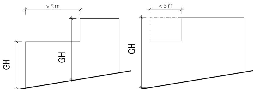
Abbildung 12: Staffelung, eigene Darstellung
