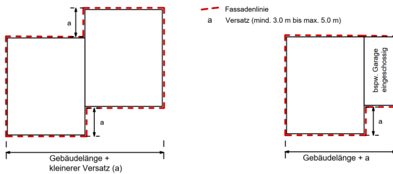
Abbildung 9: Versatz in der Situation, eigene Darstellung
