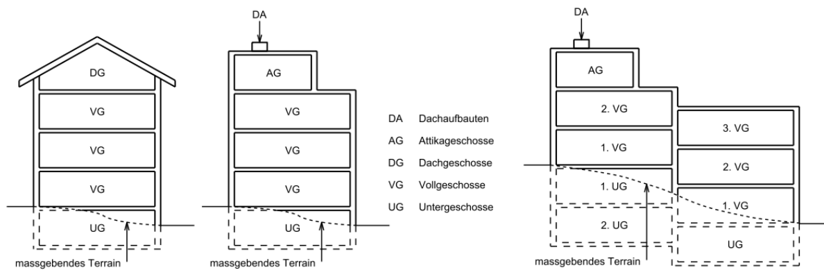
Abbildung 15: Figur 6.1 Geschosse und Geschoszahl, IVHB
