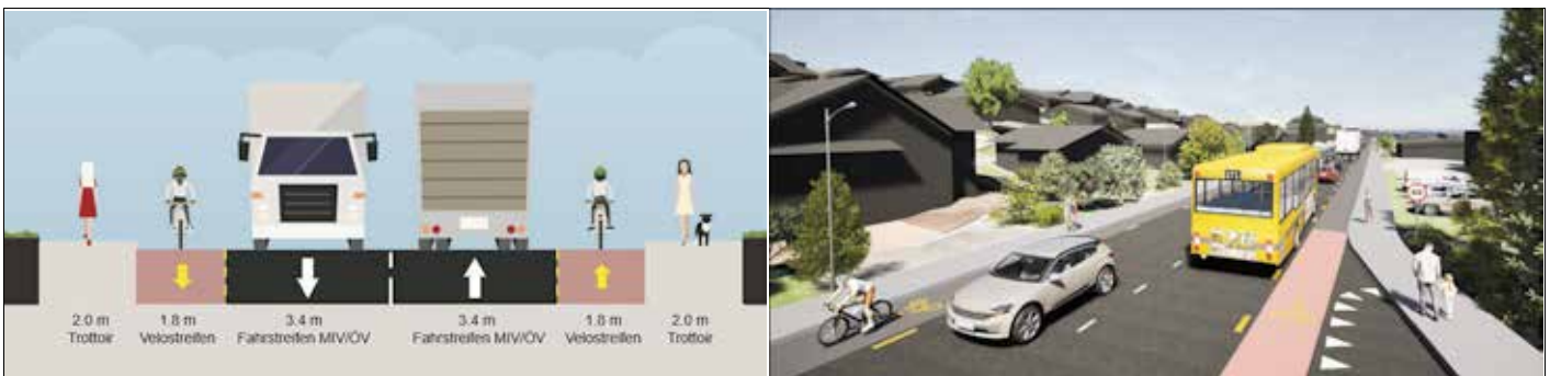
Abbildung 2: Mögliche neue Gestaltung des Strassenraums in der Variante Null+/Neugestaltung: Schötz Nord mit Radstreifen
