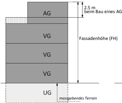
Massskizze Fassadenhöhen
