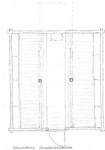
Grundriss ehemaliger Stallteil
