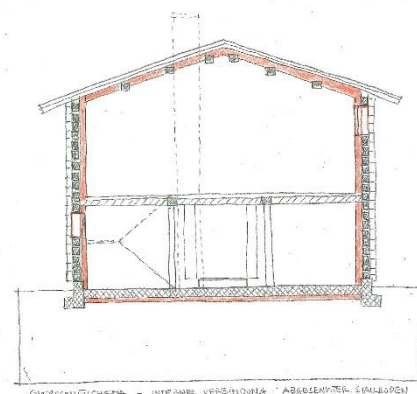
Variante 2 / Teilabbruch Heuraum, neuer Stallboden, interne Verbindung
