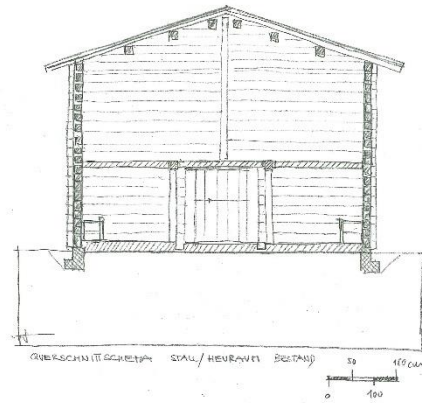
Querschnitt Heukammer/Stallteil
