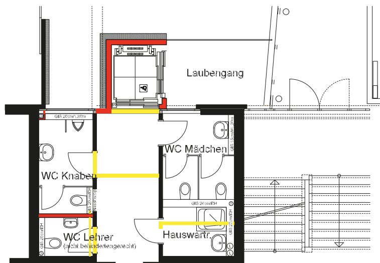
Schulhaus Grünau, Grundriss 1. Obergeschoss Nasszellensanierung/Lifteinbau
