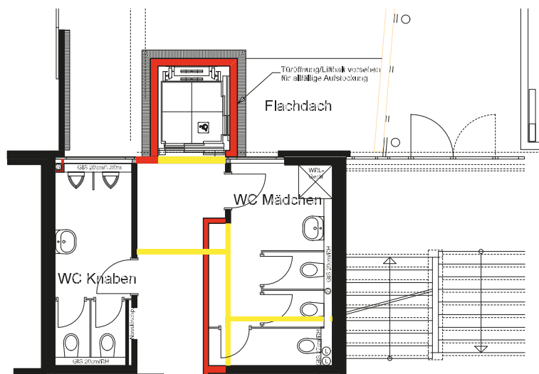
Schulhaus Grünau, Grundriss 2. Obergeschoss Nasszellensanierung/Lifteinbau
