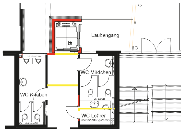
Schulhaus Grünau, Grundriss Erdgeschoss Nasszellensanierung/Lifteinbau
