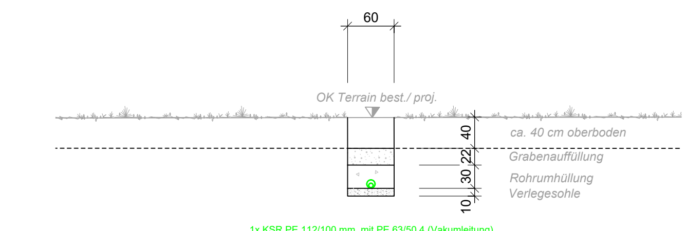
Querprofil 1 1:50
